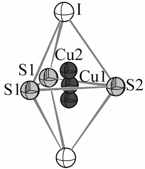
Рис. 3. Зображення мобільної катіонної підгратки для кристала \text{Cu}_6\text{AsS}_5\text{I} : тригонально-координований атом міді Cu1 знаходиться на позиції 24g, тетрагонально-координовані атоми міді Cu2 знаходяться на позиціях 48h [2].
