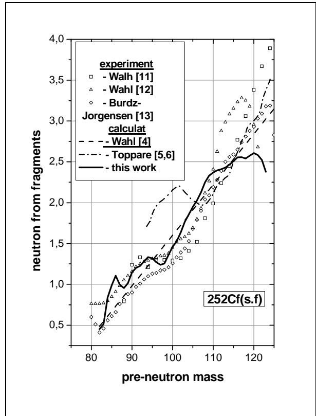
Рис.2. Залежність v_f(M) від маси первинних уламків спонтанного поділу ^{252}\text{Cf} . Квадрати, трикутники, ромби – експериментальні дані [11-13]. Лінії – результати розрахунків [4-6] та наші дані.
