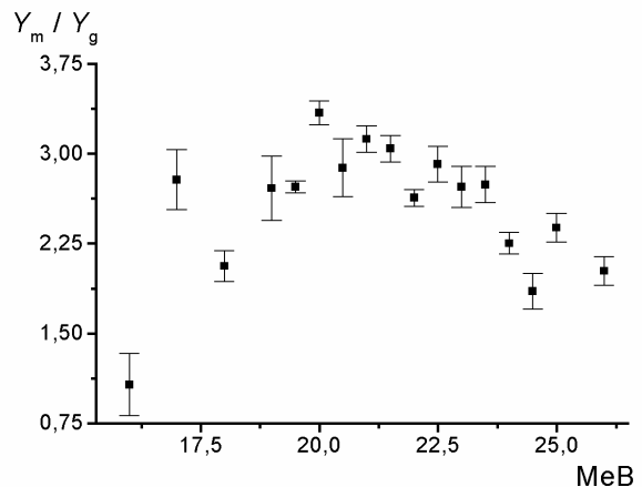
Рис. 2. Енергетична залежність ізотопних відношень для реакції ^{118}\text{Sn}(\gamma, p)^{117m,g}\text{In} .
