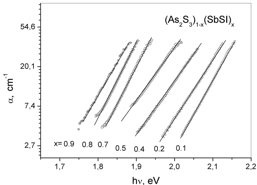
Рис.1. Спектральні залежності краю поглинання стекел (As_2S_3)_{100-x}(SbSI)_x
