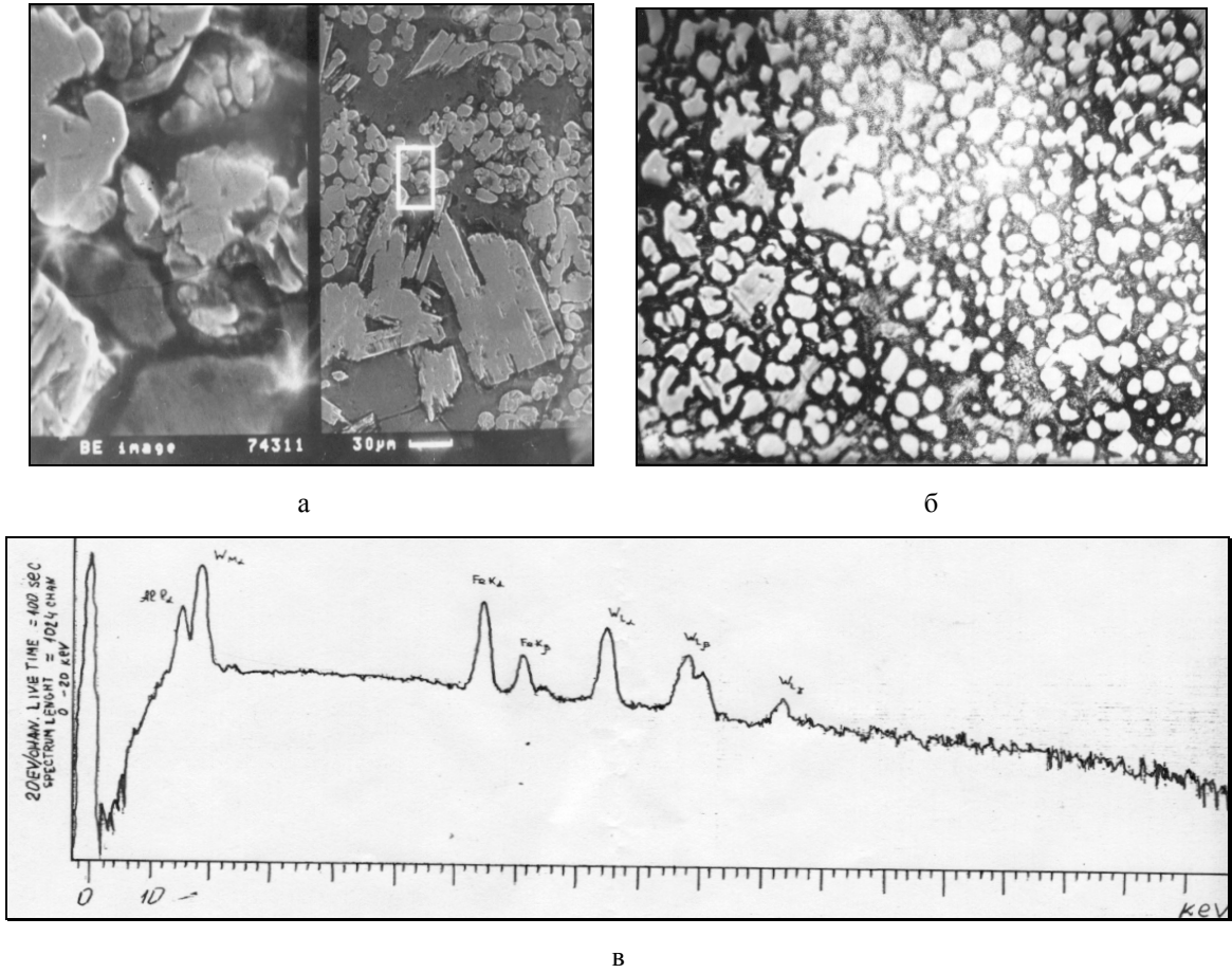
Рис. 11. Мікроструктура і рентенограма карбідосталі отриманої СВС-процесом: а, – з масивними карбідами WC в матриці швидкорізальної сталі (а – \times 1500 , \times 400 ); б – сталева матриця з глобуляризованими комплексними карбідами типу W_2C ( \times 200 ); в – рентенограма в Cu_{k\alpha} випромінюванні.
