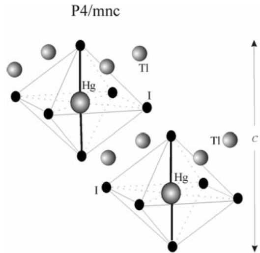
Рис. 2. Схематичне зображення кристалу Tl_4HgI_6 при температурі 296 К
