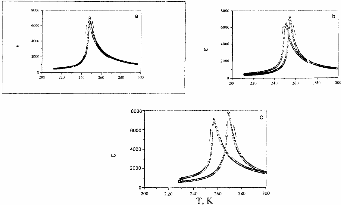
Рис.1 Температурні залежності \epsilon ( p=415 МПа, v=1 МГц) для кристала (Sn_{1-x}In_{2/3x})_2P_2S_6 , x=0.028 мол.дол. при різних швидкостях зміни температури: а- 0.8 К/хв.; б- 3.3 К/хв.; с-10 К/хв.
