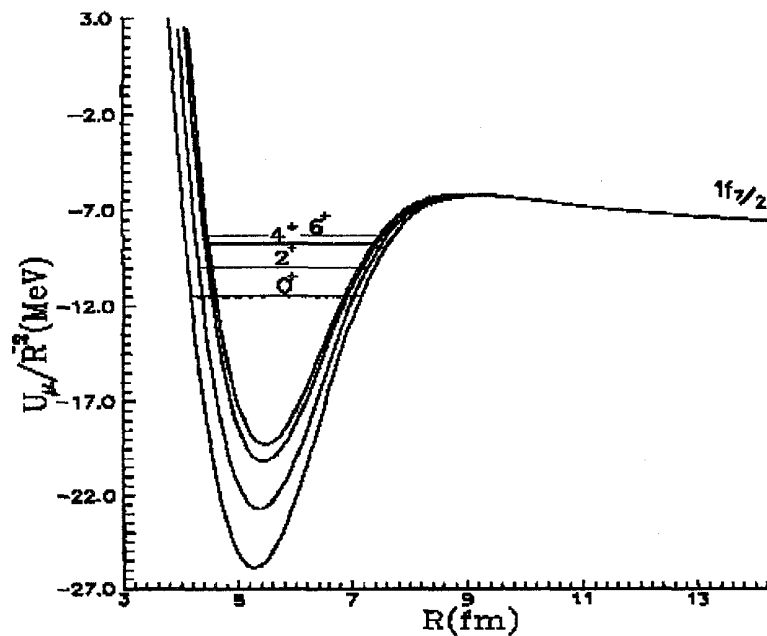
Рис. 1. Хід потенціальних кривих та їх поведінка на асимптотіці для ядра ^{42}\text{Ca} .
